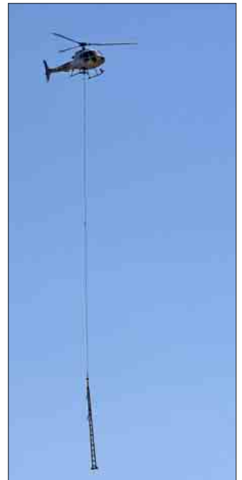
Per Hubschrauber wurden neue Oberleitungsmasten an ihren Standort transportiert und dort direkt montiert.
